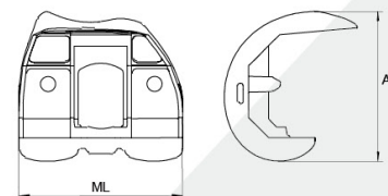
A3 Femoral Condylar (Co-Cr-Mo)
