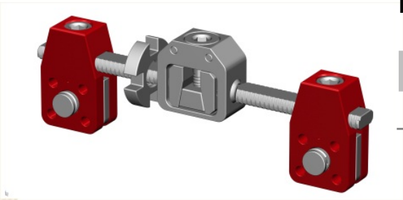
Mini Fixator - Universal
